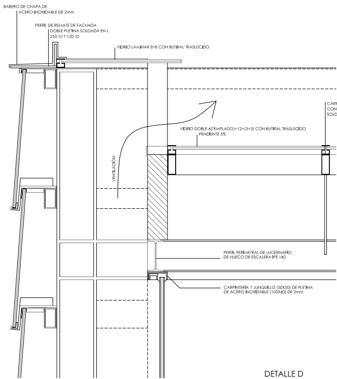
DETALLE D ENCUENTRO DE FACHADA CON CUBIERTA, LUCERNARIO DE ESCALERA
