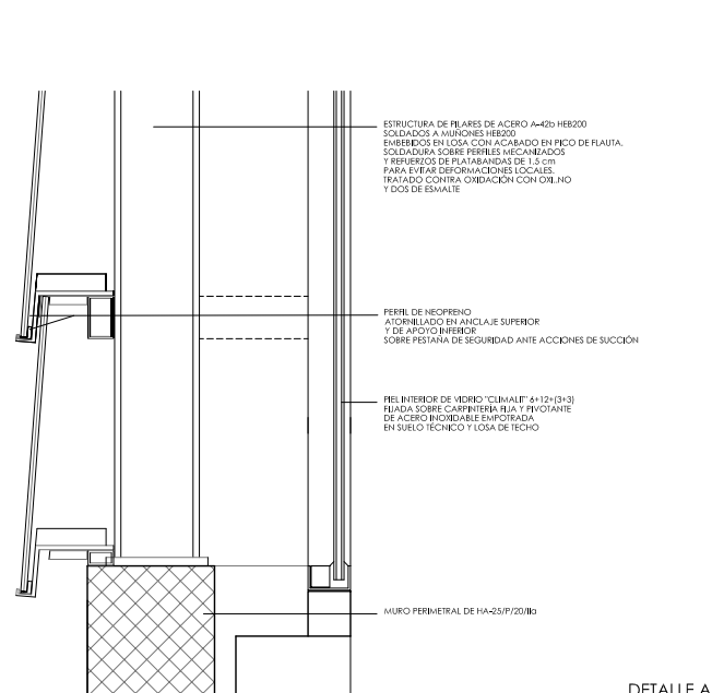
DETALLE A ARRANQUE DE FACHADA DESDE MURO DE HORMIGON
