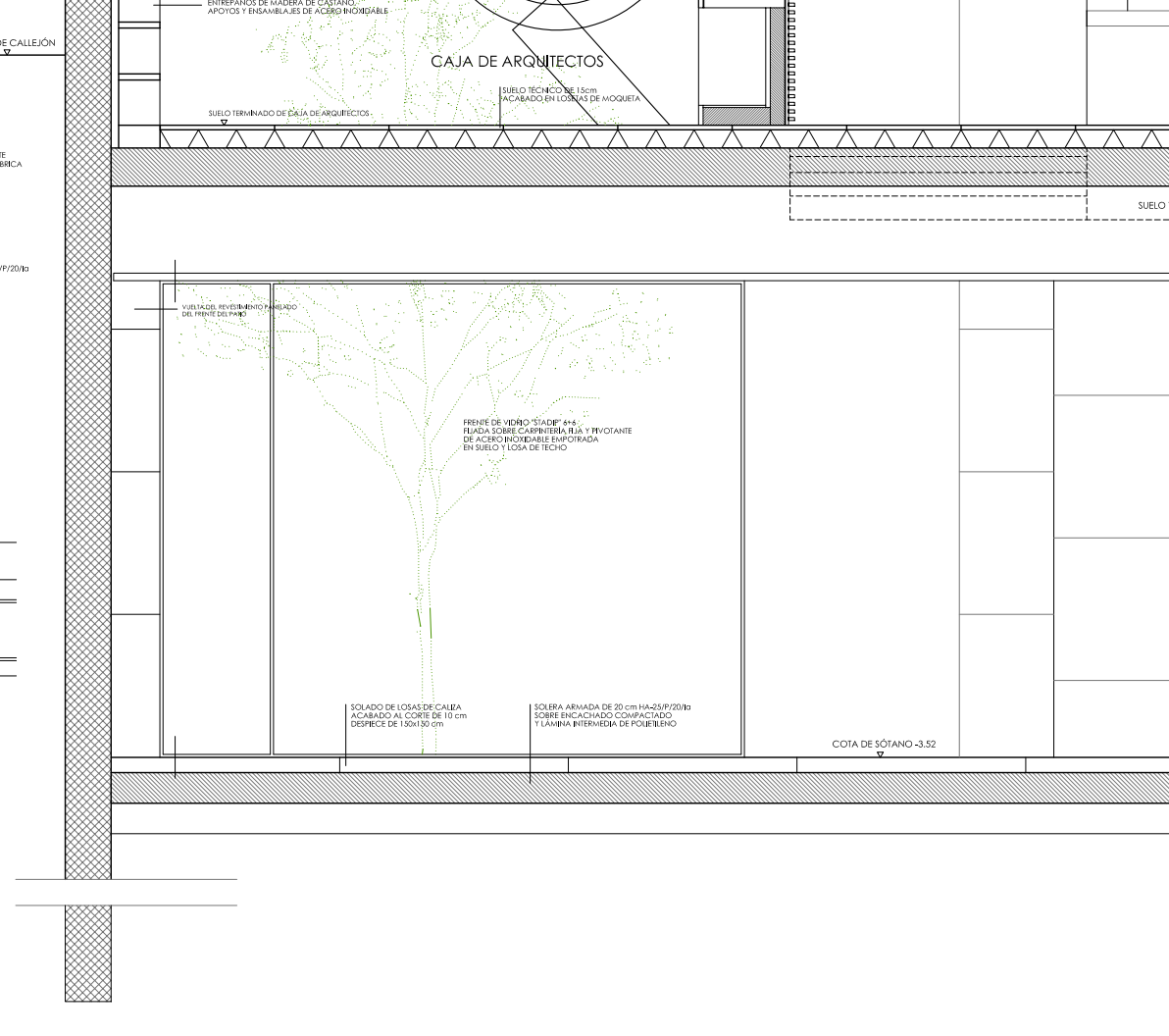
DETALLES CERRAMIENTO LATERAL Y POSTERIOR
