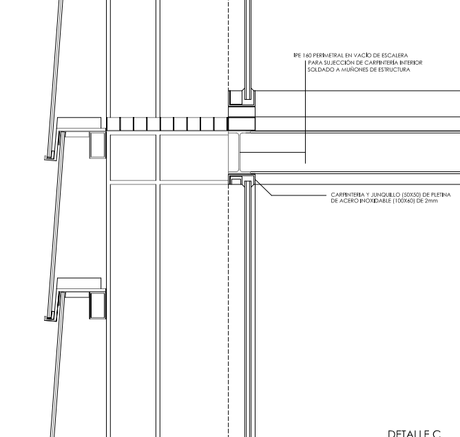
DETALLE C ARRANQUE DE FACHADA DESDE MURO DE HORMIGON
